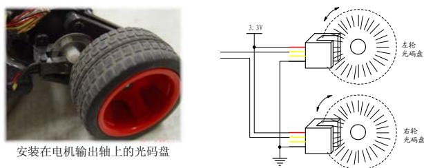
图 6- 7 采集电机光电码盘信号
