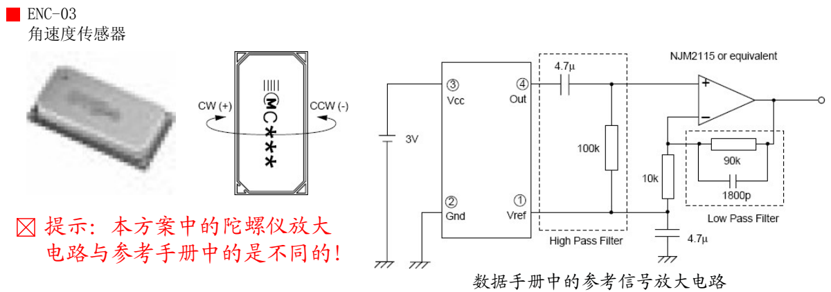
图 2- 19 角速度传感器及参考放大电路
