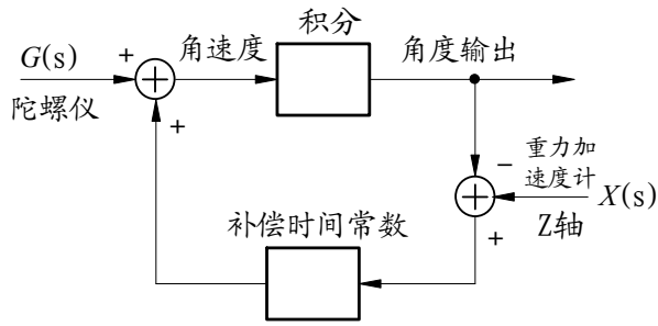
图 3-22 角度计算环节的传递函数
