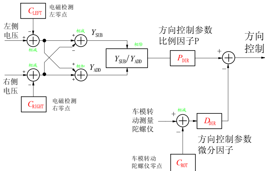
图 2- 39 车模方向控制算法
